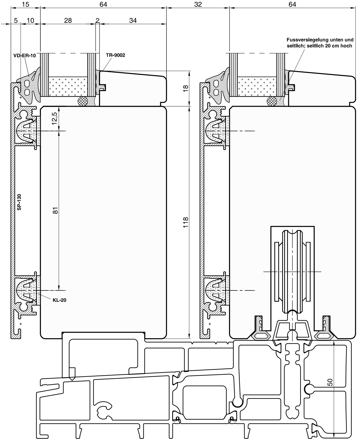
Siegenia Bodenschwelle HH7642-06 A0069 inkl. Laufschiene HH0131-04
